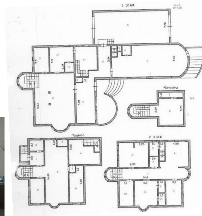
Схем-план
