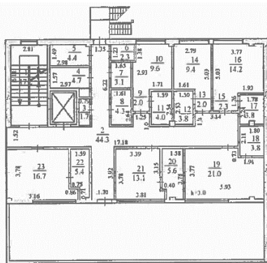
4 этаж
